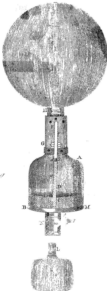
Fig. 1. Sea Gauge.
